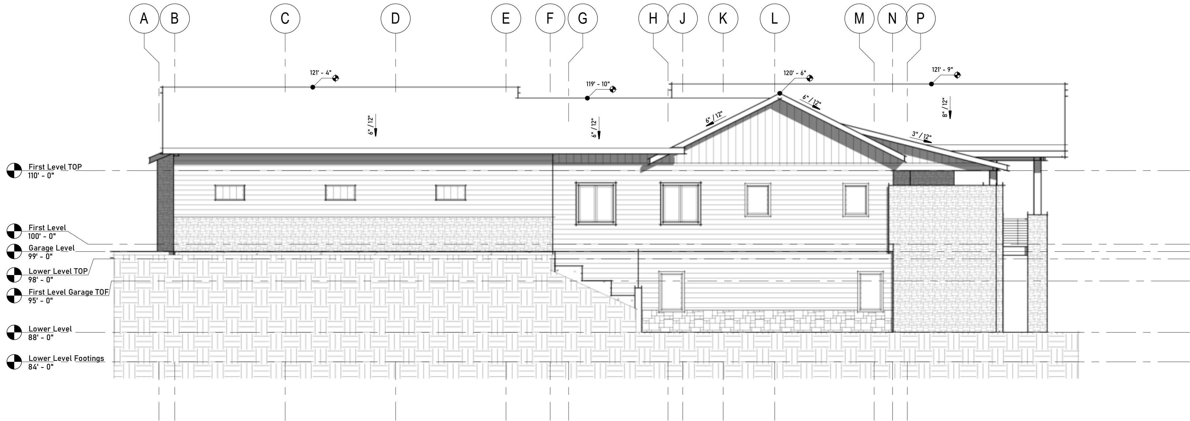
A3 Side Exterior Elevation 1 Scale: 1/8" = 1'-0"
