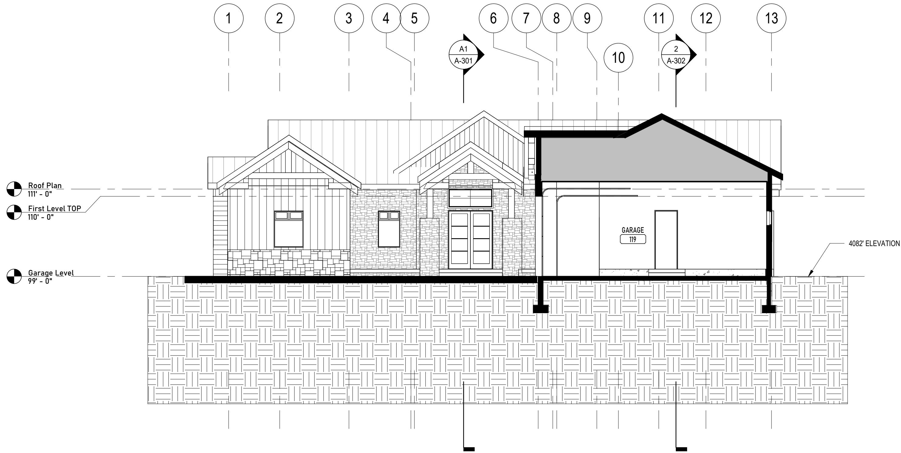
A3 Section 2 Scale: 1/8" = 1'-0"
