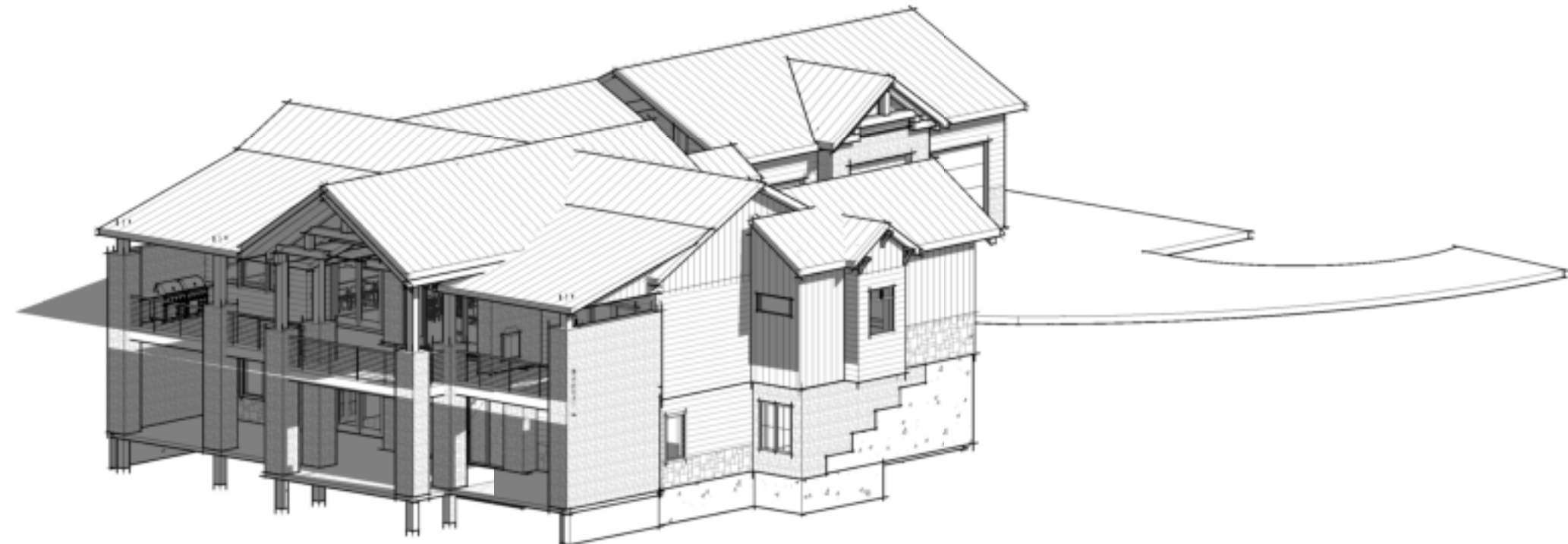
A3 Front View 2 Scale:
