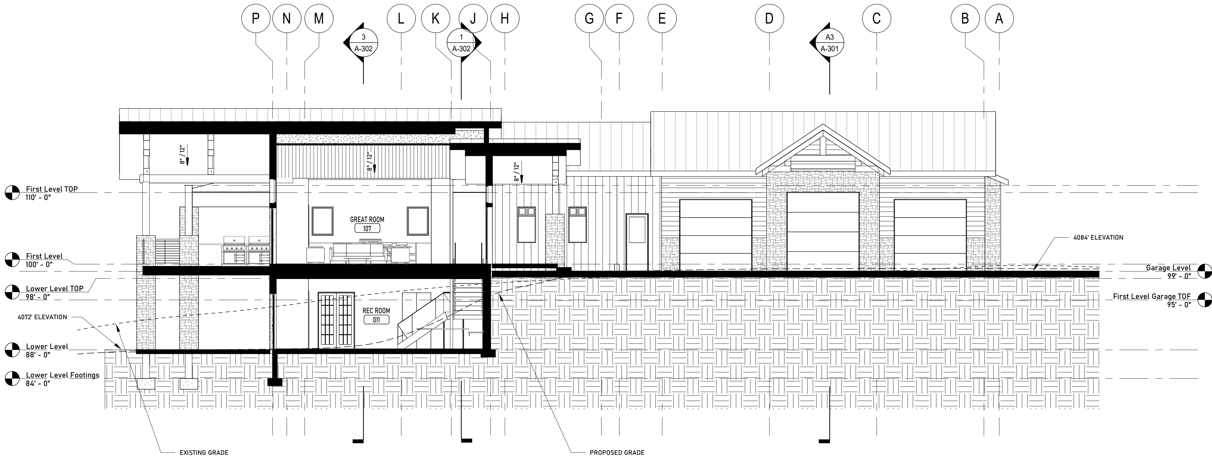
A1 Section 1 Scale: 1/8" = 1'-0"
